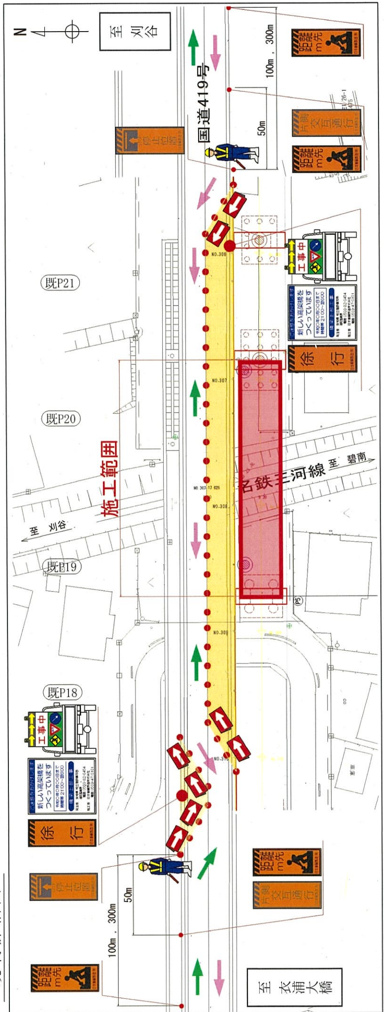
規制詳細図
